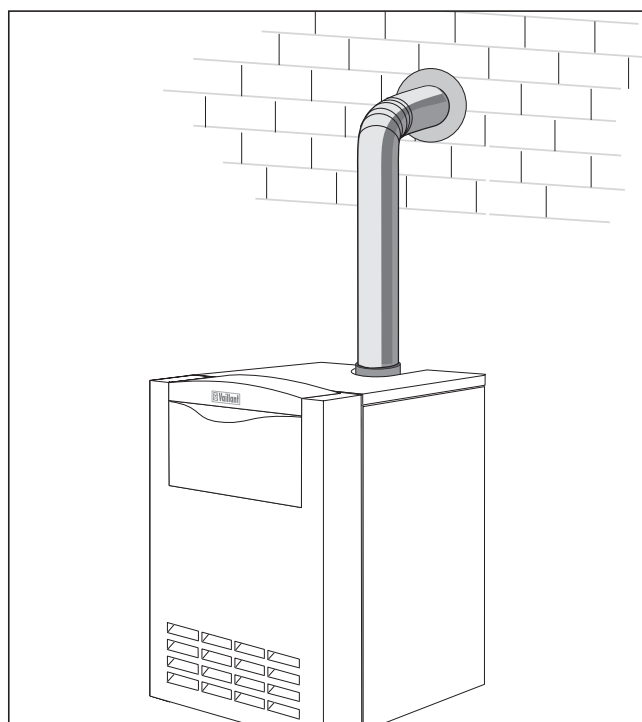
Sl. 4.3 Montaža nastavkov izpušnih plinov
