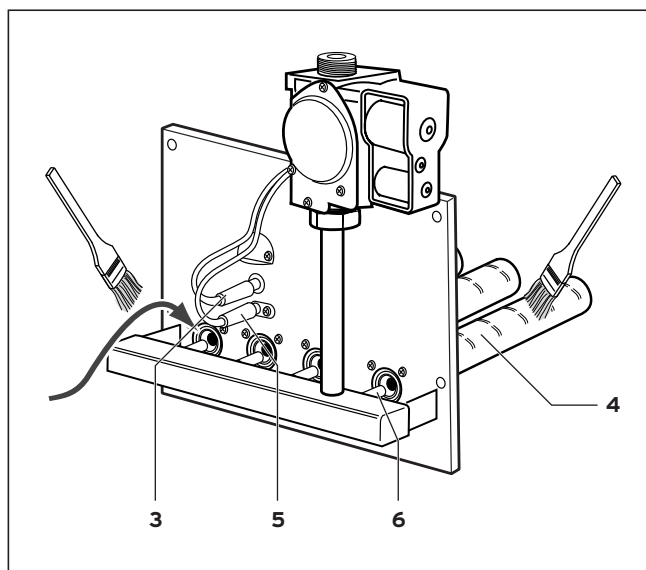
Sl. 7.3 Čiščenje gorilnika
