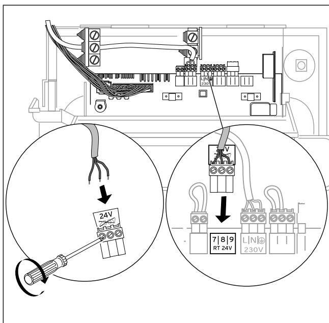
Fig. 4.7 Conectarea regulatorului la 7-8-9
