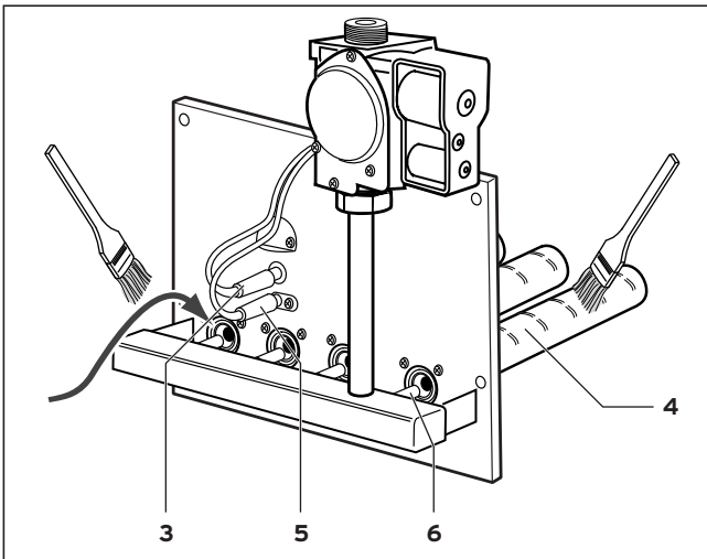
Fig. 7.3 Curățarea arzătorului
