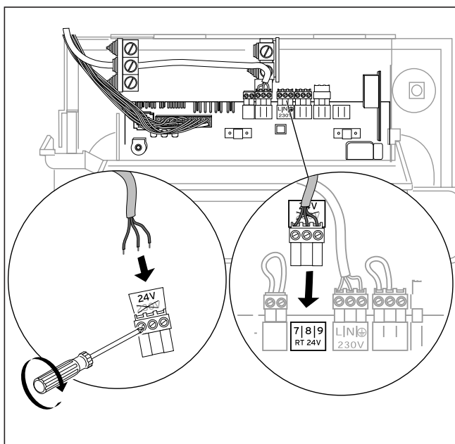
Sl. 4.7 Priključiti regulator na stezaljke 7-8-9
