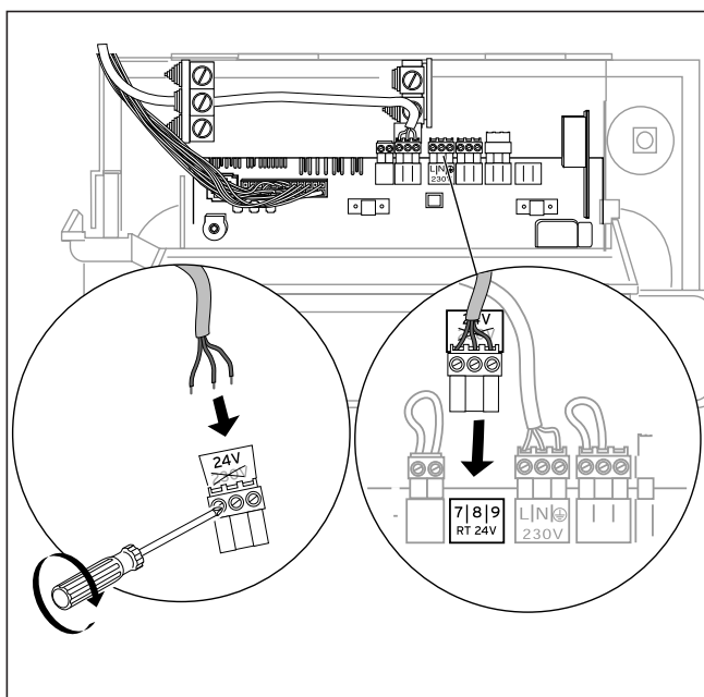
Sl. 4.7 Temperaturni regulator priklopimo na sponke 7-8-9
