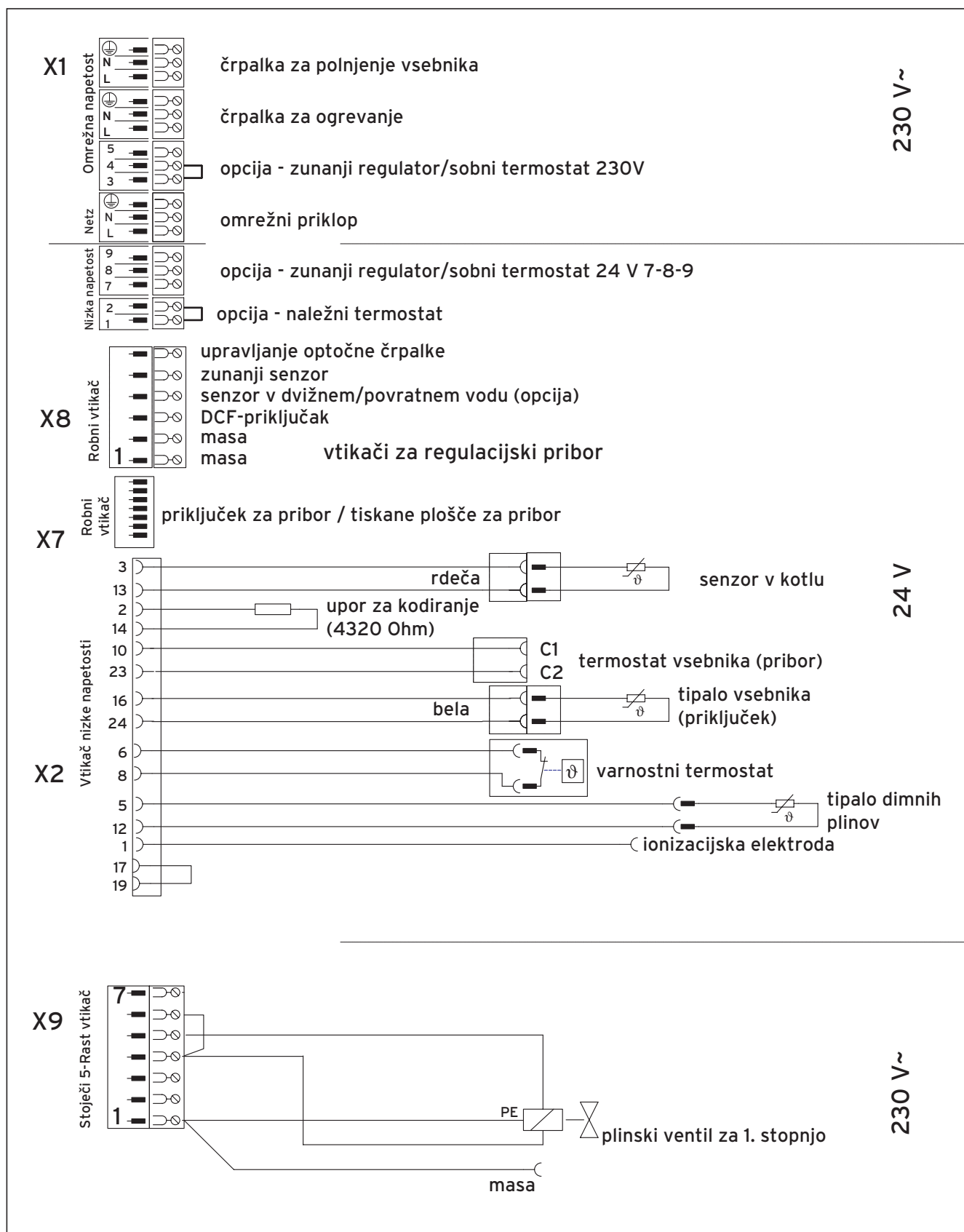
SI. 4.5 Električni priključki atmoVIT
