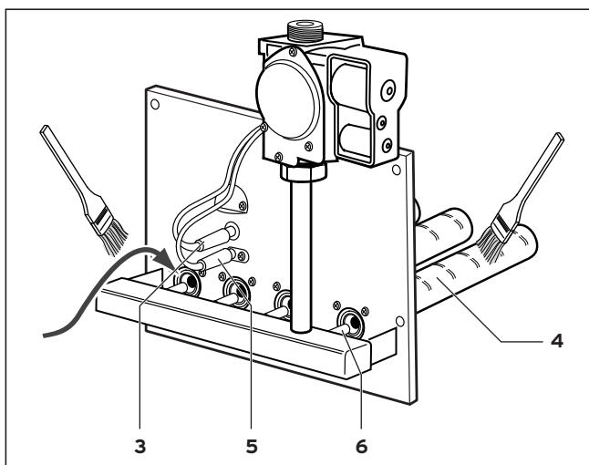
Slika 7.3 Čišćenje plamenika
