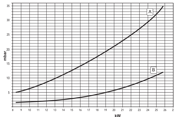
fig. 18 - Diagramă presiune - putere
