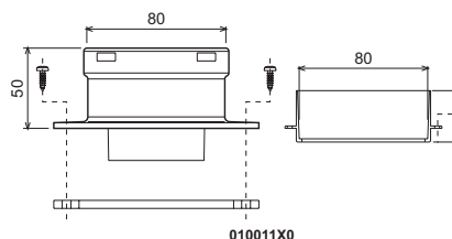
fig. 12 - Accesoriu de plecare pentru conducte separate
