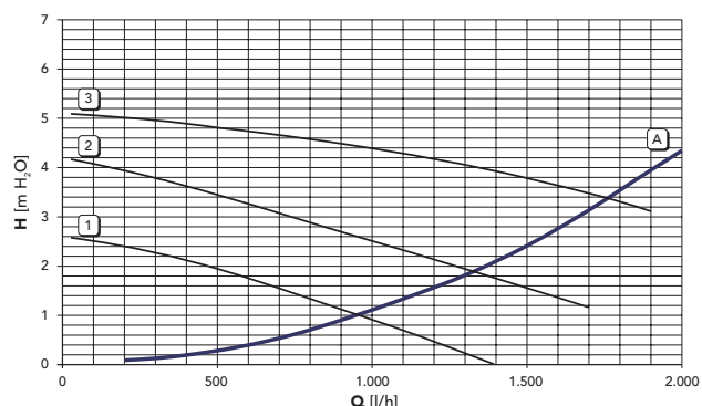
fig. 19 - Pierderi de sarcină / înălțime de pompare pompe de circulație DOMIproject F 24 D
