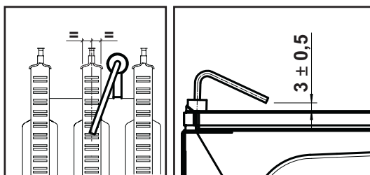
fig. 16 - Poziționarea electrodului
